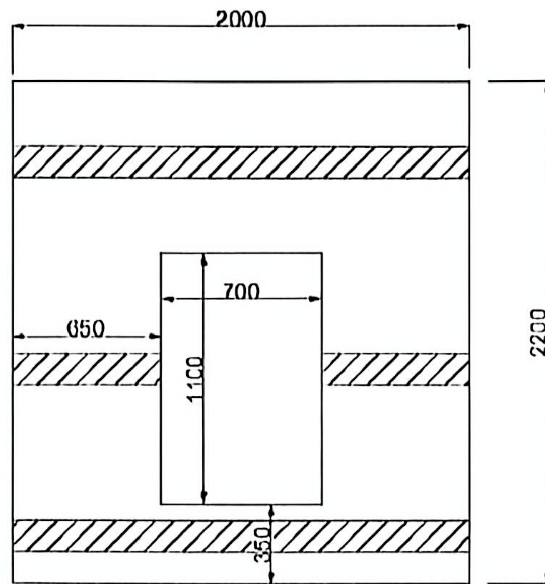
风门示意图
